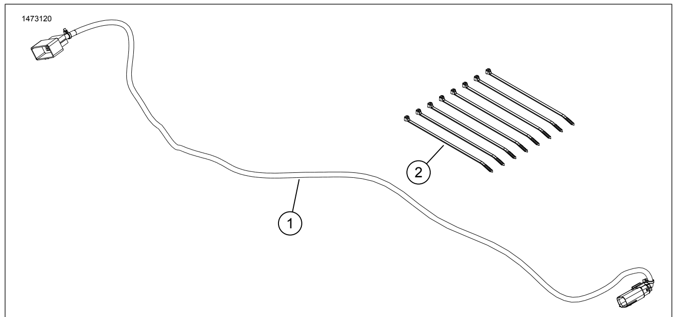
Figur 3. Servicedelar, installationssats för förstärkare
