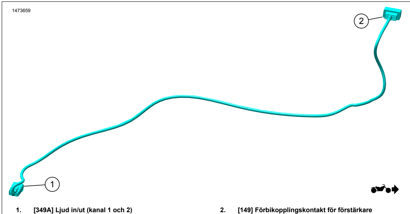
Figur 1. Kablage till kåphögtalare
