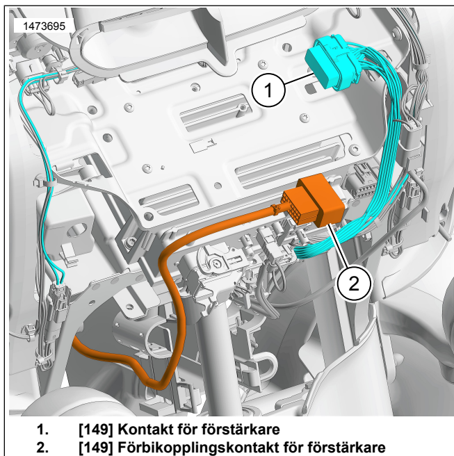
Figur 2. Gaffelmonterad kåpa visas, fast kåpa likartad
