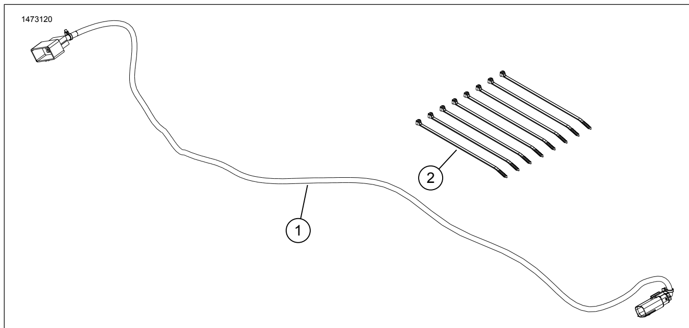
Figure 3. Mga Pamalit na Piyesa, Kit sa Pagkakabit ng Amplifier
