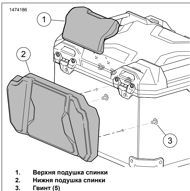
Малюнок 4. Установіть спинку
