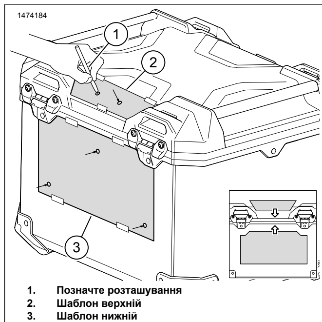
Малюнок 2. Розташування шаблонів
