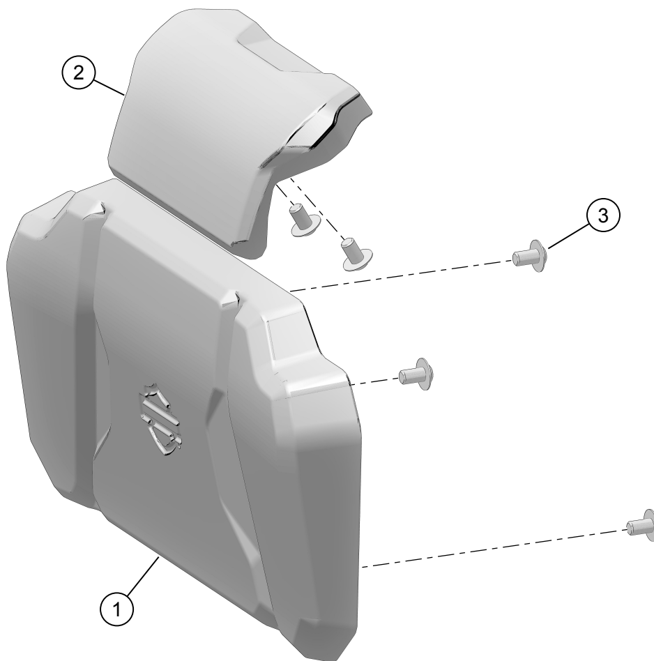
Малюнок 1. Вміст комплекту: Спинка
