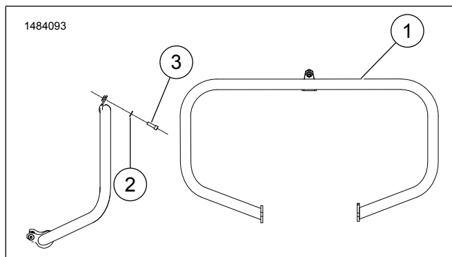
图1。维修零件：发动机护罩套件
