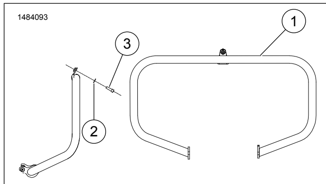
圖1。維修零件引擎護蓋組
