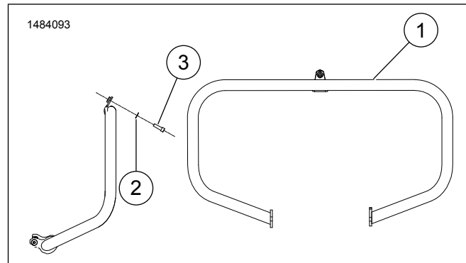
Slika 1. Servisni dijelovi: Komplet štitnika motora
