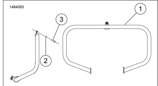
Εικόνα 1. Ανταλλακτικά: Κιτ προστατευτικού κινητήρα
