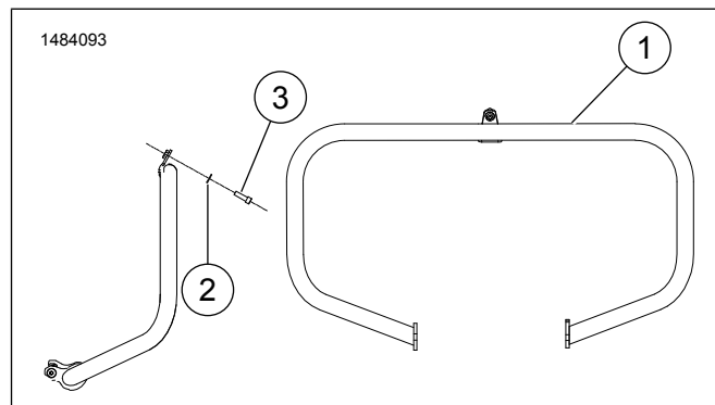
図1. 交換用パーツ: エンジンガードキット
