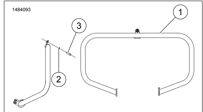
Pav 1. Dalys, reikalingos užduočiai atlikti Variklio apsaugos rinkinys
