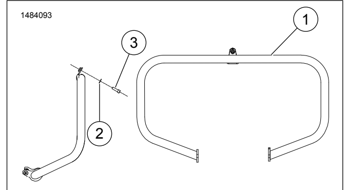
Rajah 1. Bahagian Servis: Kit Adang Enjin
