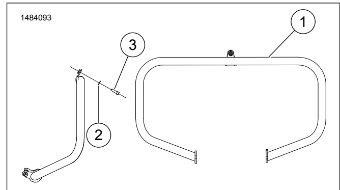
Rysunek 1. Elementy zestawu serwisowego: Zestaw osłony silnika
