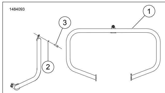
Obrázok 1. Servisné diely: Súprava padacieho rámu motora
