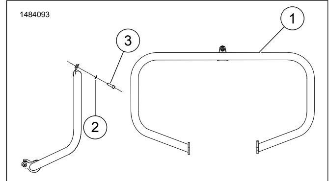
Figura 1. Piezas de servicio: Kit de protector del motor
