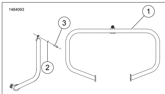
รูปภาพ 1 อะไหล่สำรอง: ชุดแผงป้องกันเครื่องยนต์
