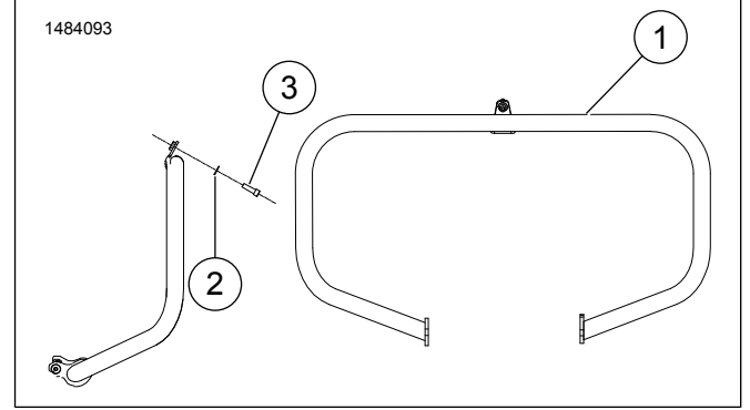
Şekil 1. Servis Parçaları: Motor Koruyucusu Kiti
