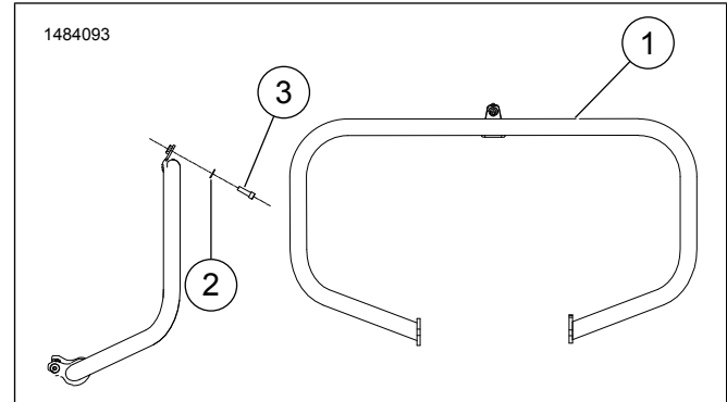
Малюнок 1. Запчастини, що обслуговуються: Комплект захисного кожуха двигуна
