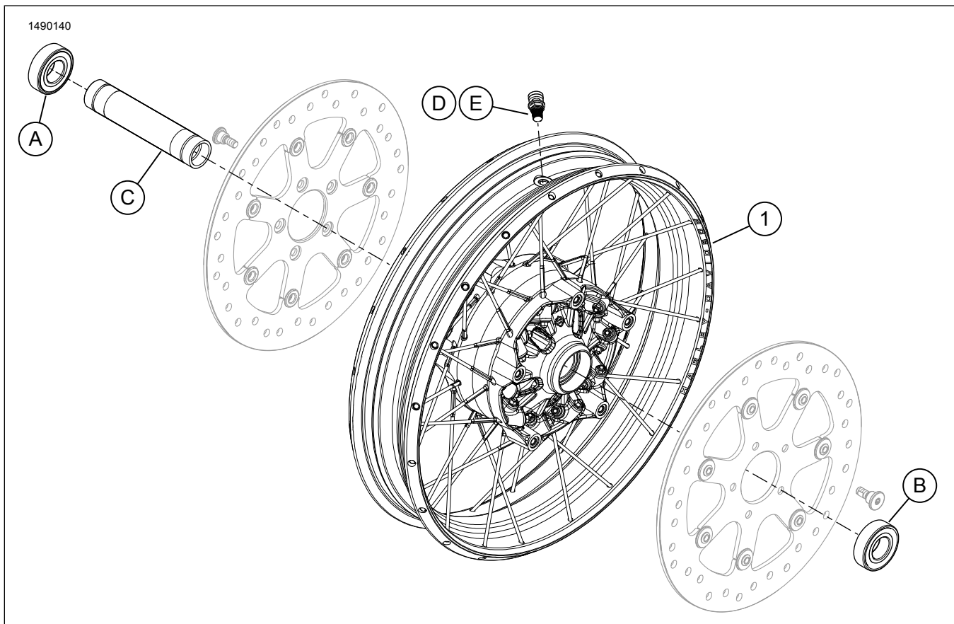
Figure 1. Pièces de rechange : Kit de roue avant
