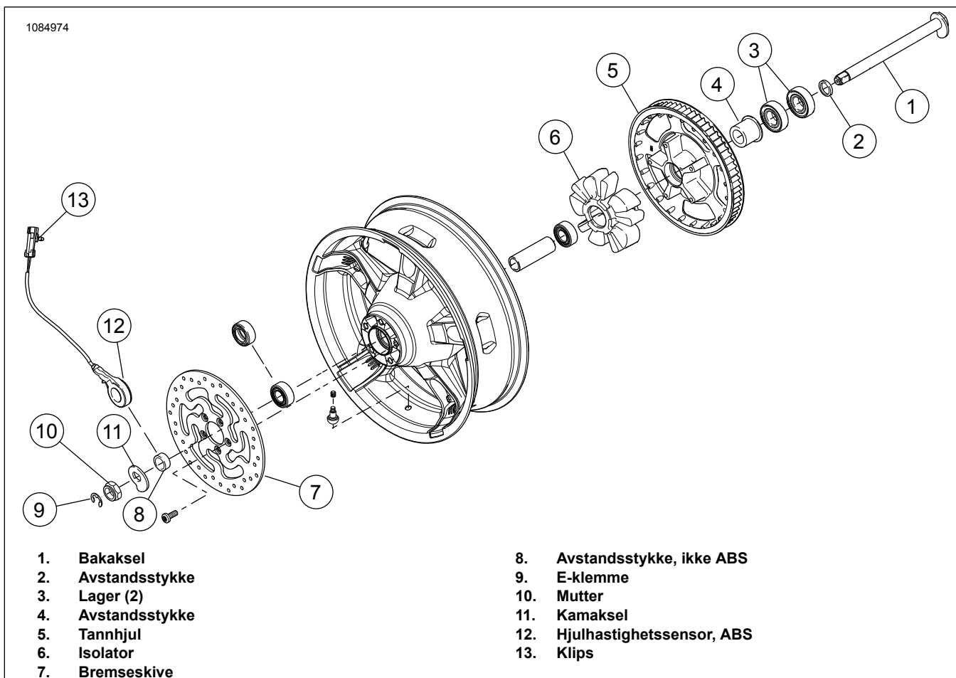
Figur 5. Bakhjulsdelar for gjenbruk
