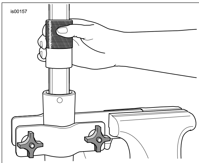
Figur 7. Montera gaffeloljaätning
