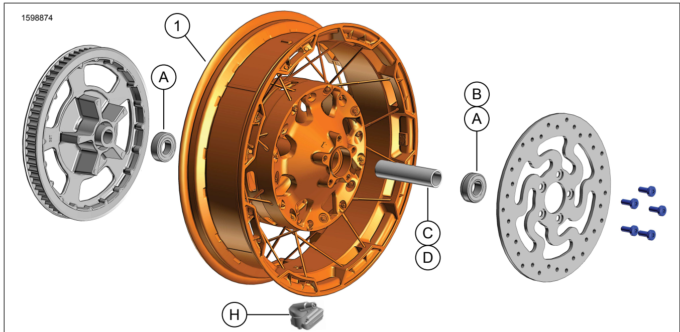
Obrázok 1. Obsah súpravy: Zadné koleso
