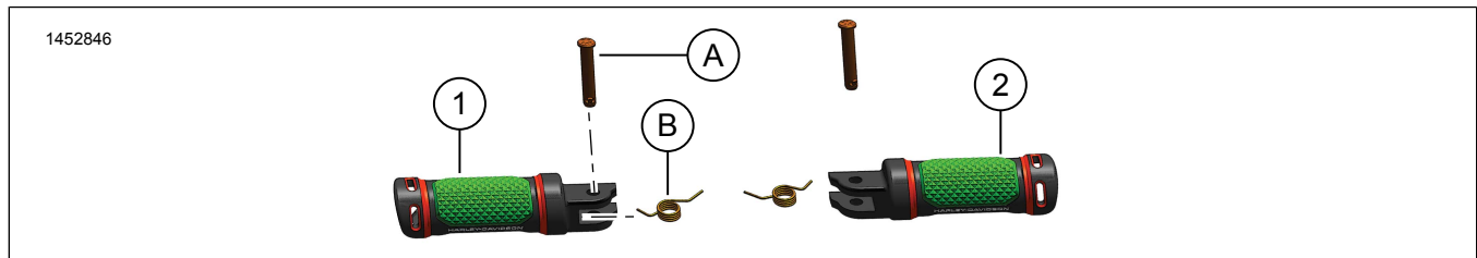
Фигура 1. Съдържание на комплекта: Стъпенки Aggressive Edge - Водач
