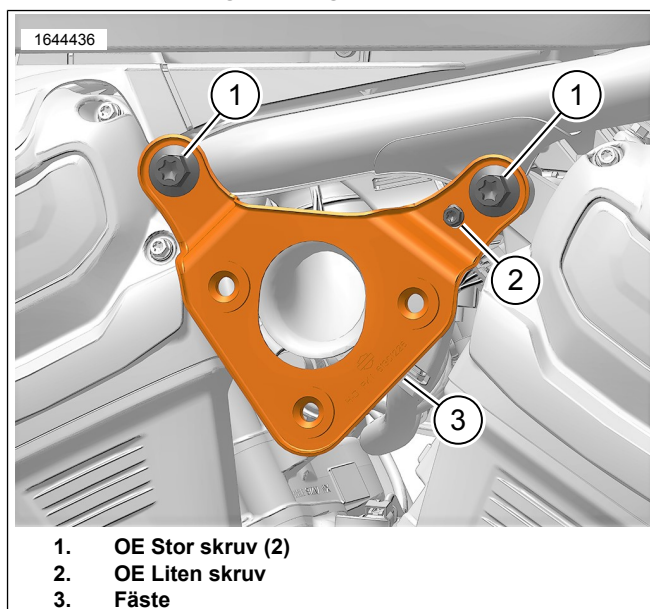
Figur 3. Fäste
