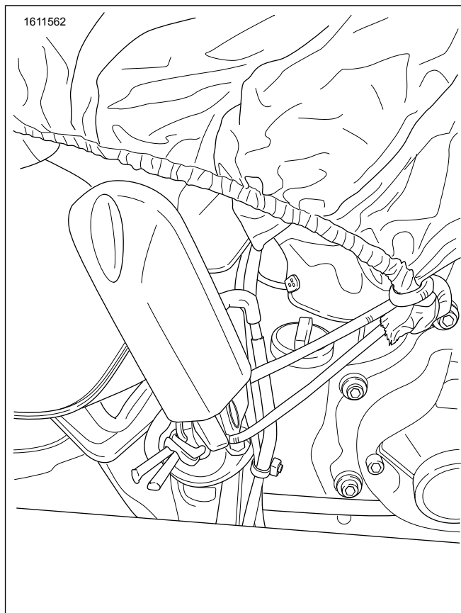
Figure 10. Fixation du marche-pied
