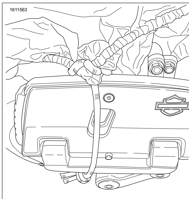
Figure 11. Fixation de plancher
