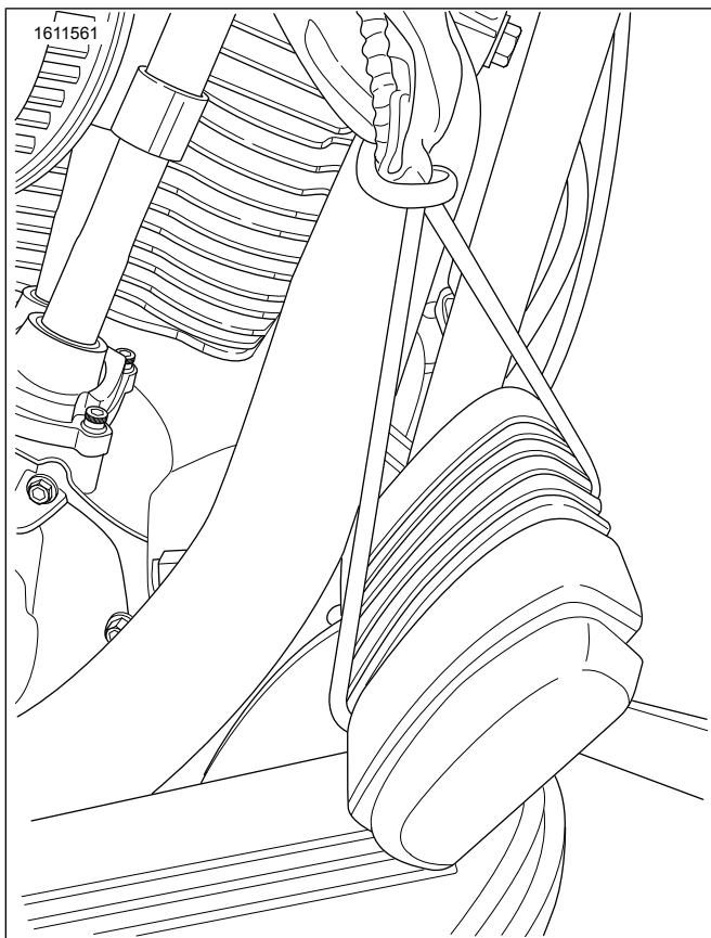
Figure 8. Fixation de la pédale de frein
