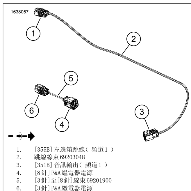
圖 16。跳線線束
