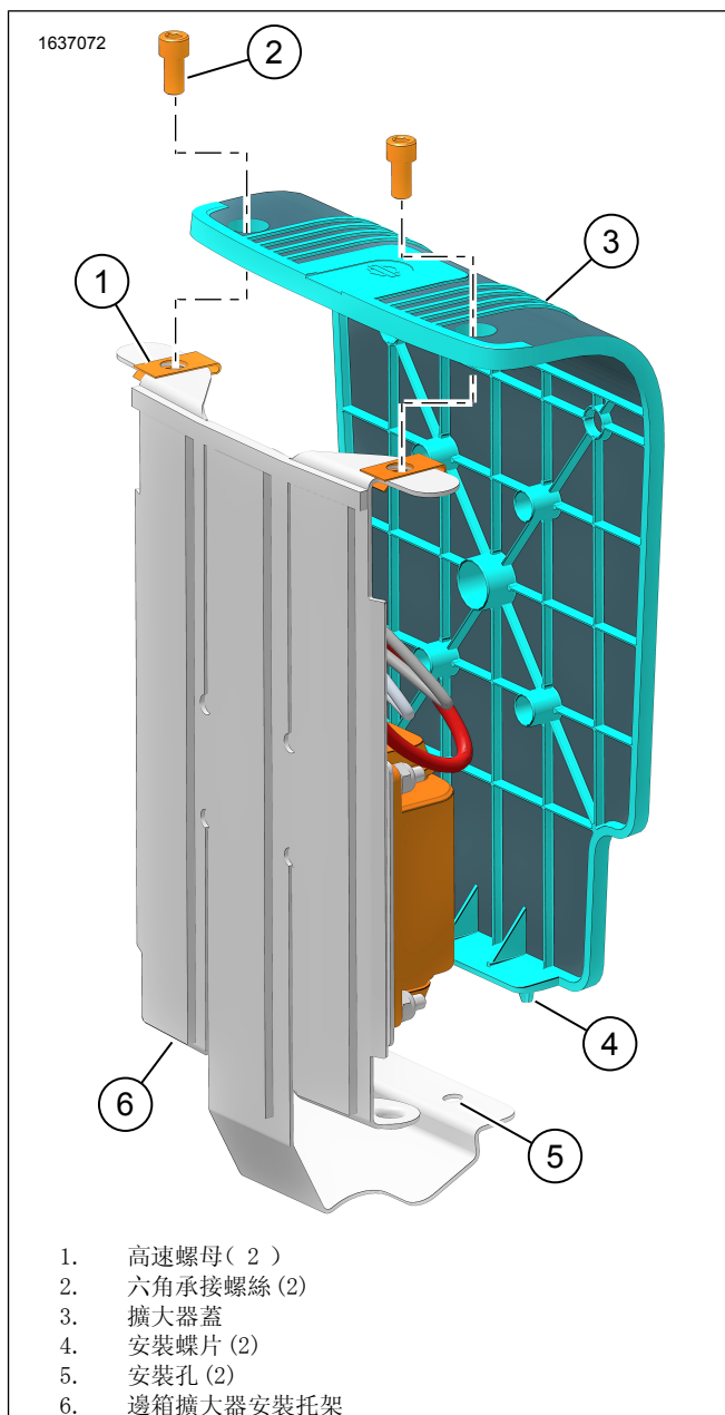
圖14。擴大器蓋
