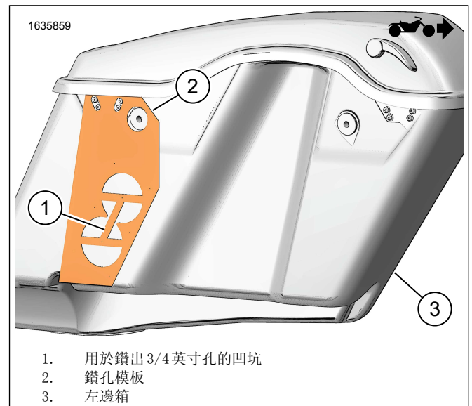
圖3。左側邊箱
