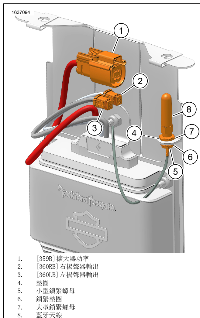
圖10。擴音器組件
