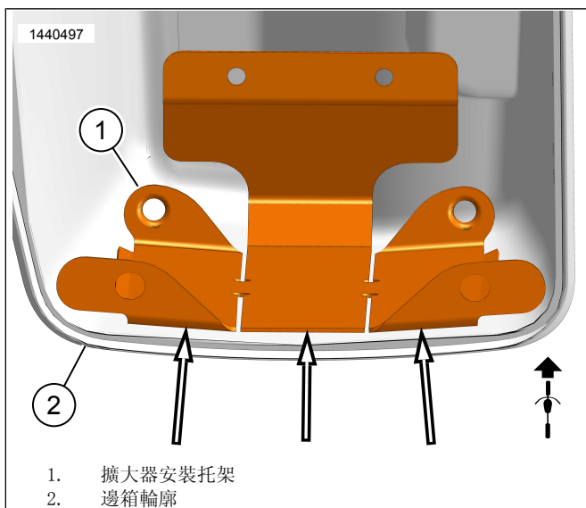
圖12。邊箱輪廓
