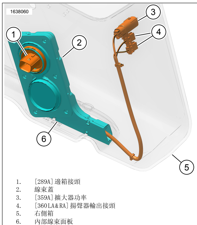
圖8。內部線束 69202871
