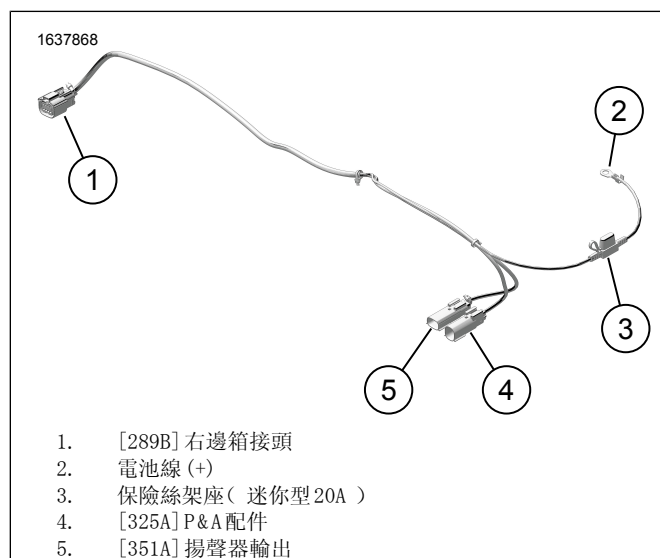
圖 15。外部線束 69202870
