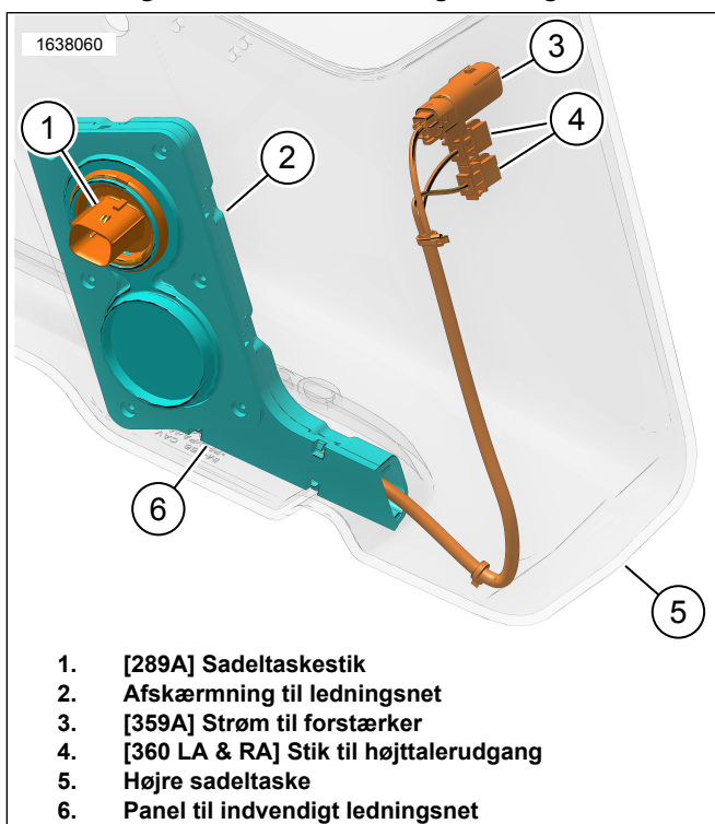
Figur 8. Indvendigt ledningsnet 69202871
