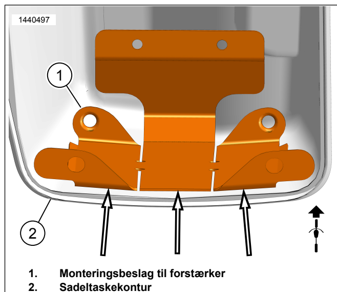
Figur 12. Sadeltaskekontur
