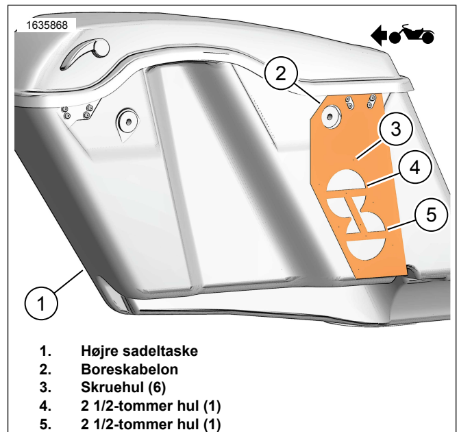
Figur 2. Højre sadeltaske
