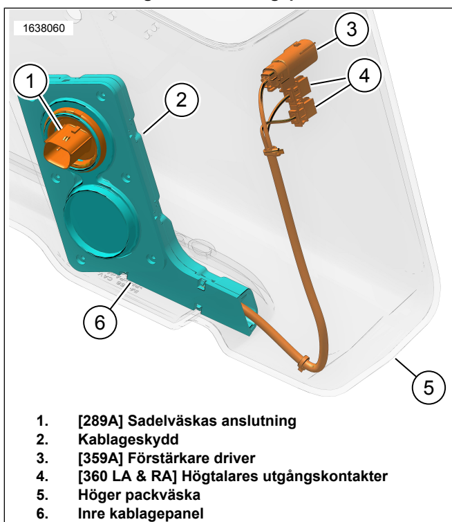
Figur 8. Inre ledningskablage
