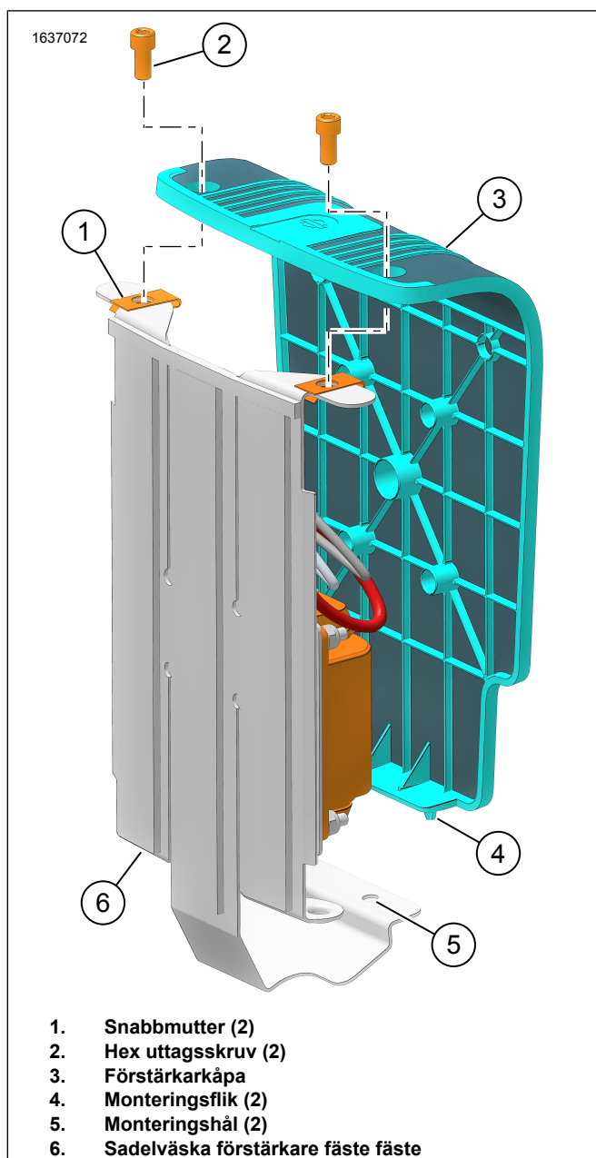
Figur 14. Förstärkarkåpa
