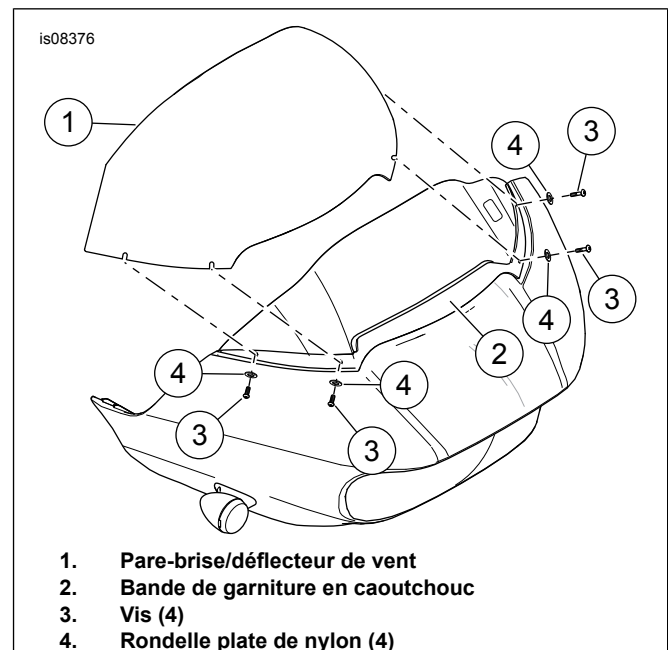
Figure 1. Installation du pare-brise / déflecteur de vent
