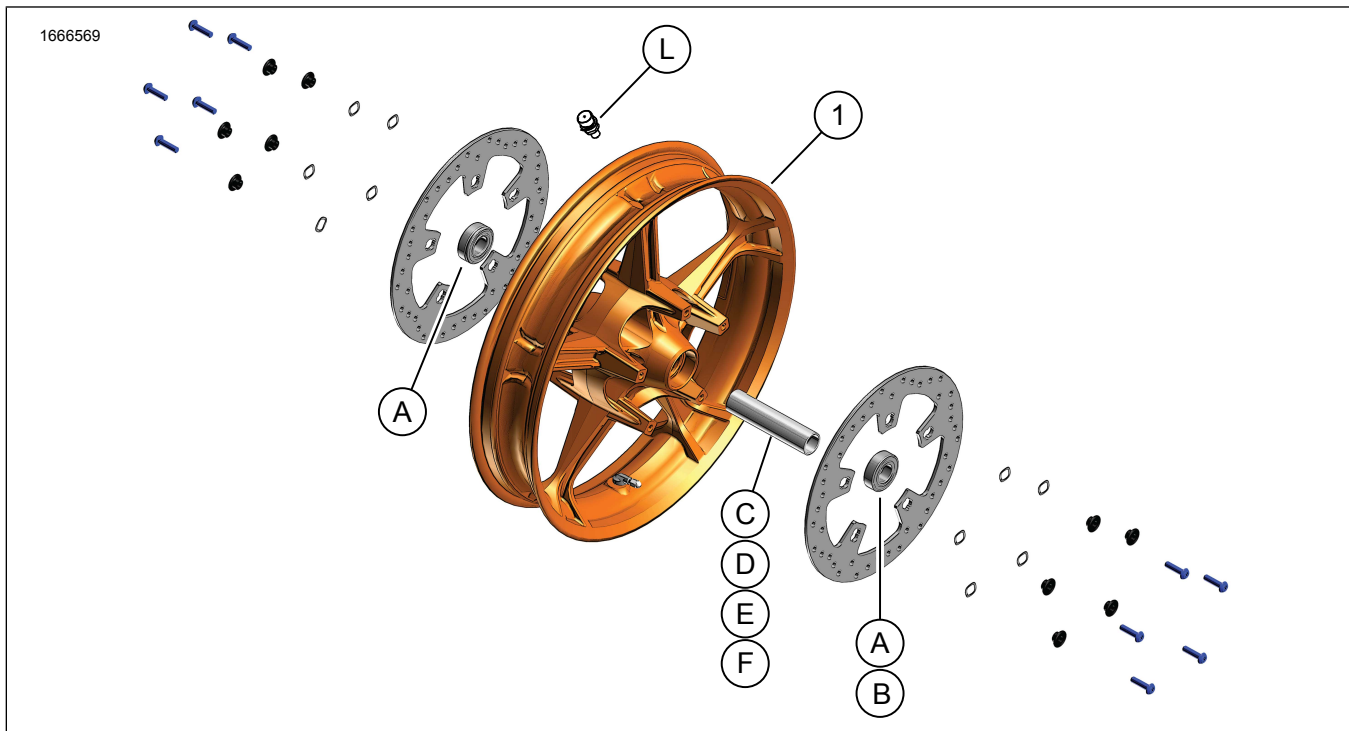
Afbeelding 1. Serviceonderdelen: Voorwiel
