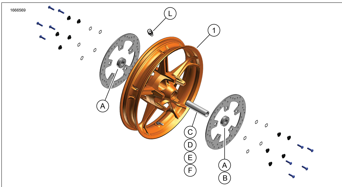
Ábra 1. Szervizelhető alkatrészek: Első kerék
