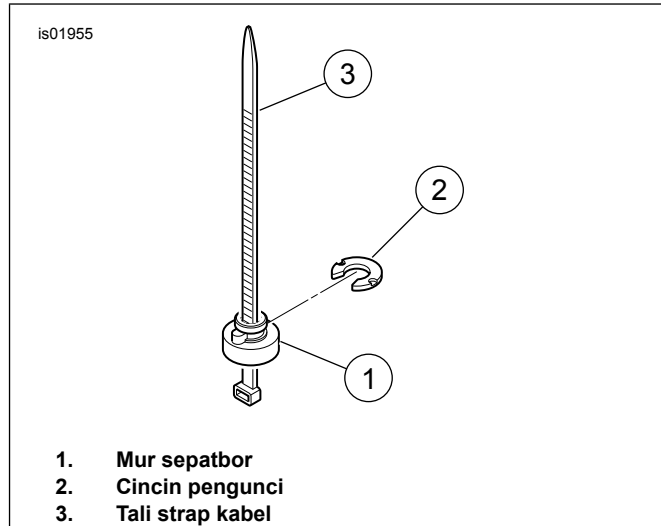
Gambar 2. Pasang mur Sepatbor
