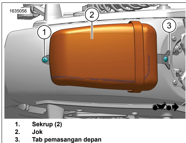
Gambar 5. Pasang Sadel Penumpang
