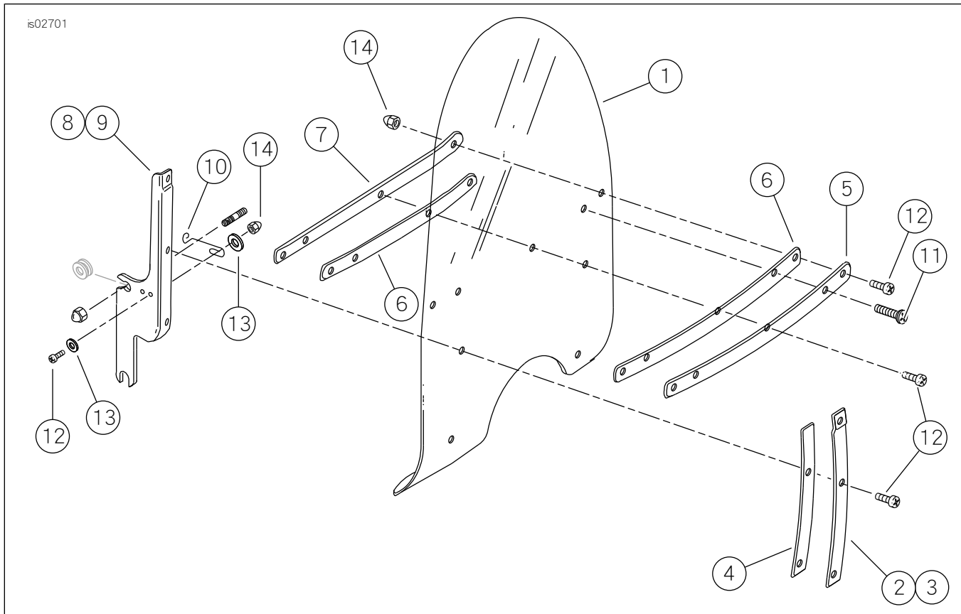
圖1。維修零件FLHR擋風玻璃工具包(國際)
