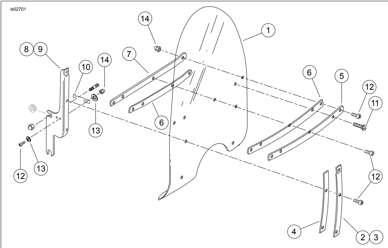
รูปภาพ 1 อะไหล่สำรอง: ชุดอุปกรณ์กระบอกกันลมรุ่น FLHR (ตลาดระหว่างประเทศ)
