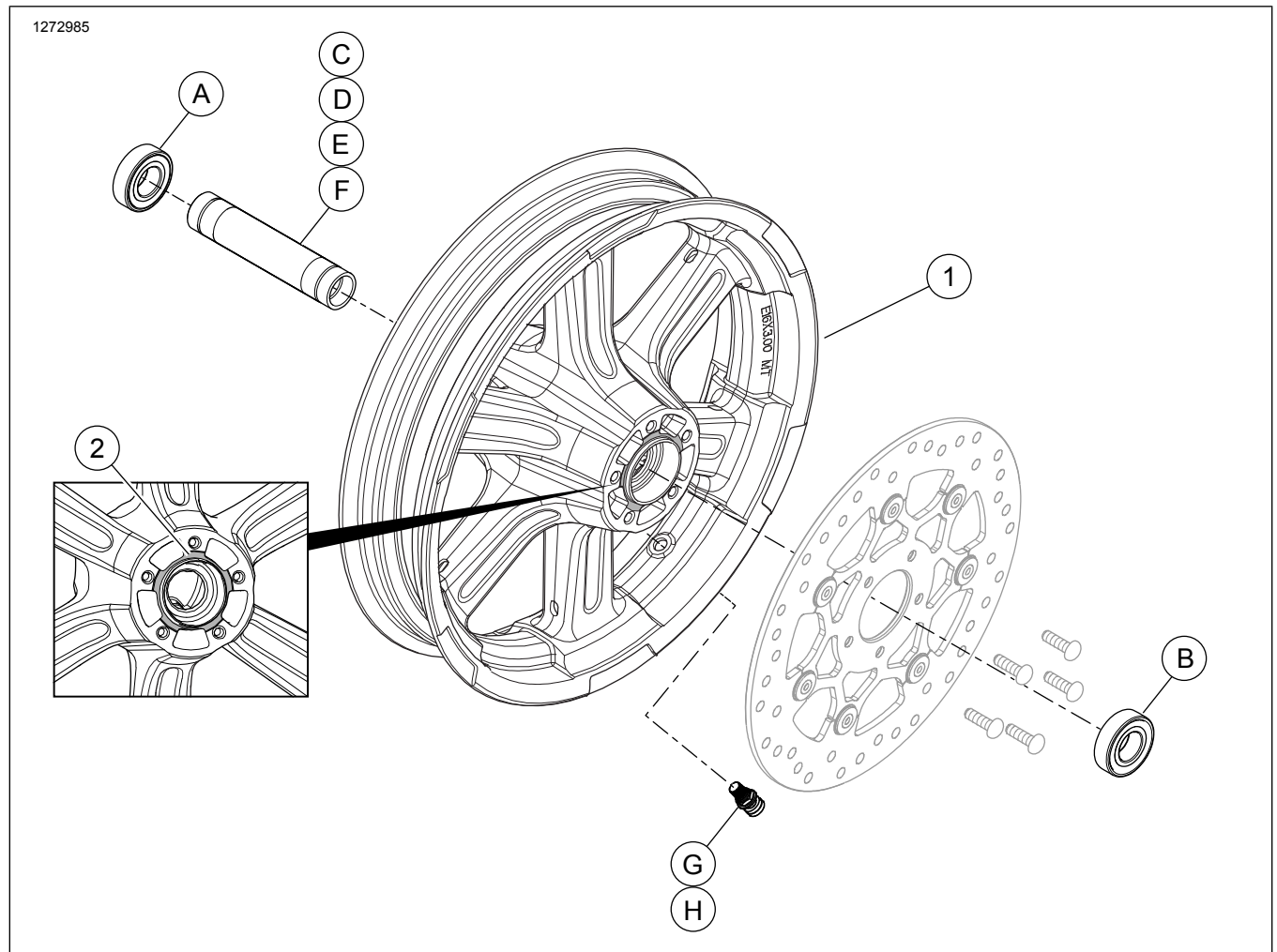
Hình 2. Phụ tùng: Bộ mâm trước
