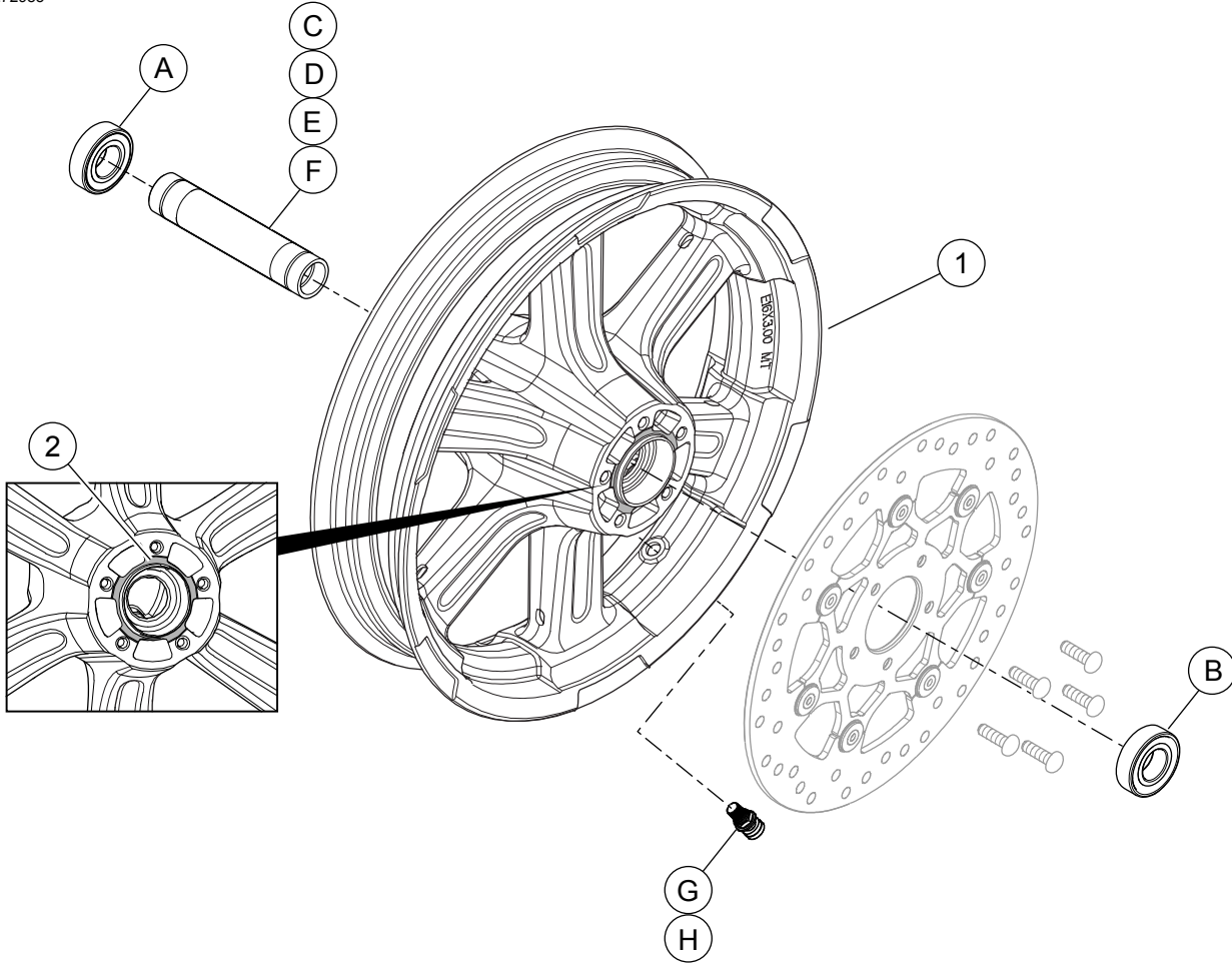
الشكل 2. قطع غيار الخدمة: مجموعة العجلة الأمامية
