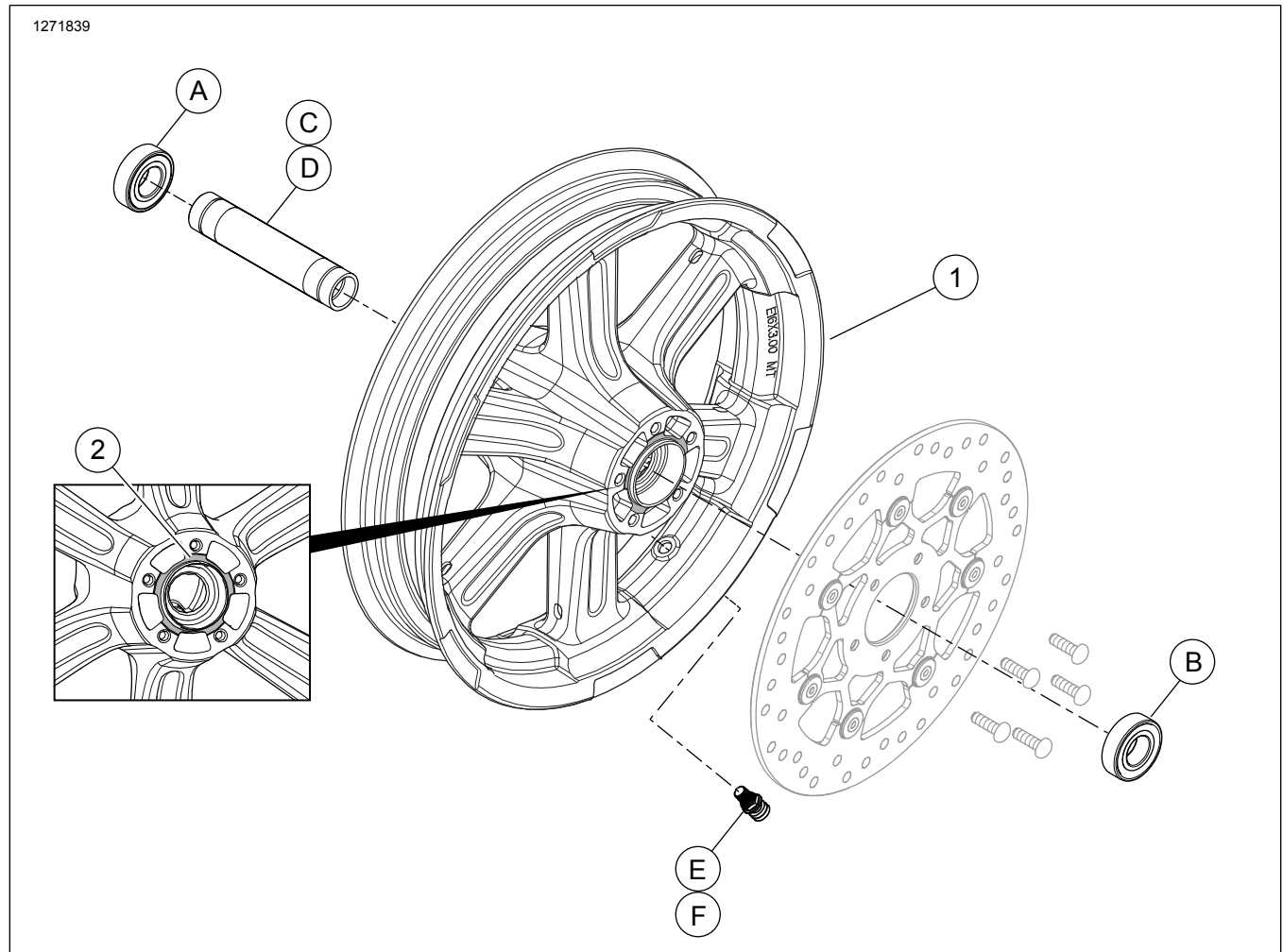
Afbeelding 1. Serviceonderdelen: Achterwiel (16 inch afgebeeld)
