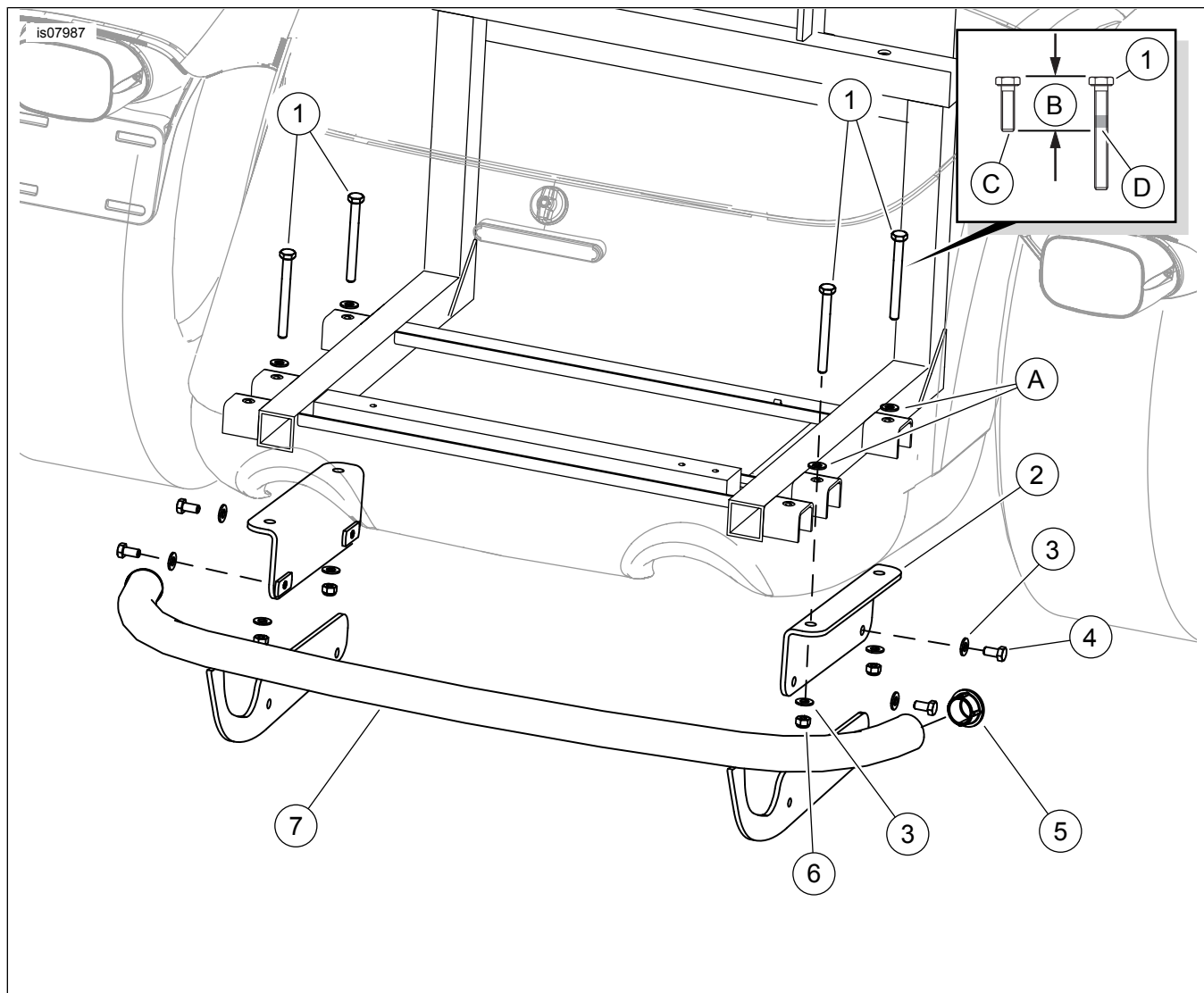
รูปภาพ 1 อะไหล่สำรอง: ชุดแผงป้องกันด้านหลังสโคอร์เมียม Trike
