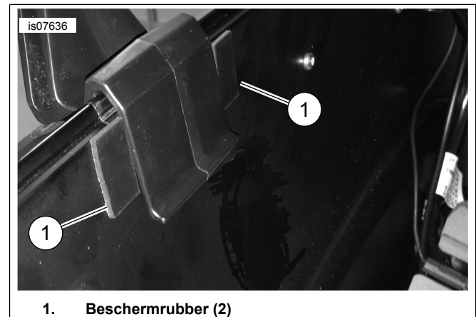
Afbeelding 2. Monteer beschermrubbers aan de binnenzijde van de Tour-Pak
