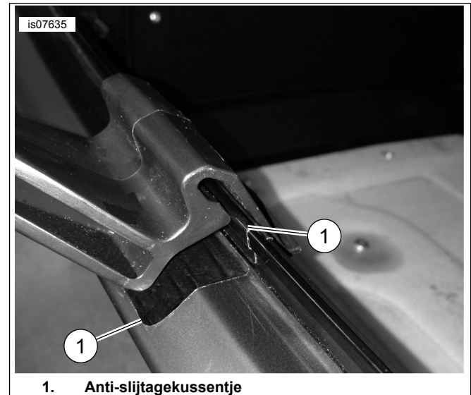
Afbeelding 1. Monteer een anti-slijtagekussentje op de Tour-Pak
