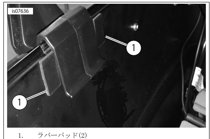
図2. ツアーパックの内側へのラバーパッドの取付
