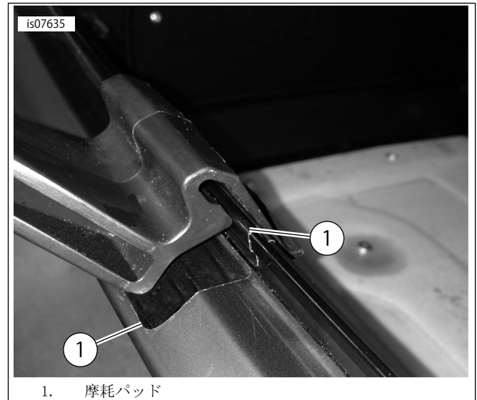
図1. ツアーパックへの摩耗パッドの取付
