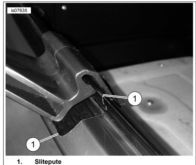
Figur 1. Monter sliteputen på Tour-Pak
