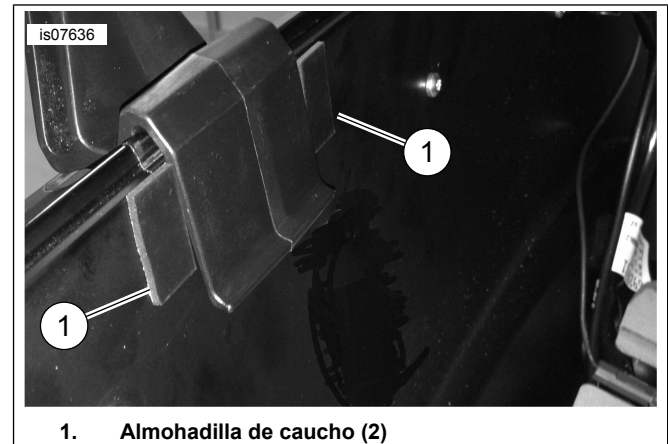
Figura 2. Instale las almohadillas de caucho en el interior del Tour-Pak.
