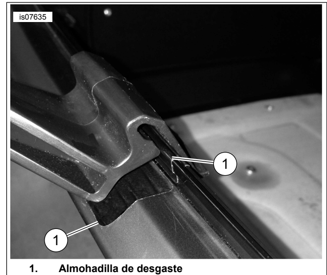
Figura 1. Instale la almohadilla de desgaste en el Tour-Pak
