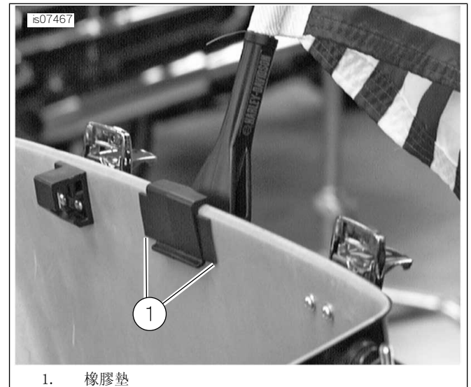
圖2。安裝在Tour-Pak內部的橡膠墊
