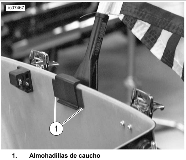
Figura 2. Almohadillas de caucho instaladas en el interior del Tour-Pak
