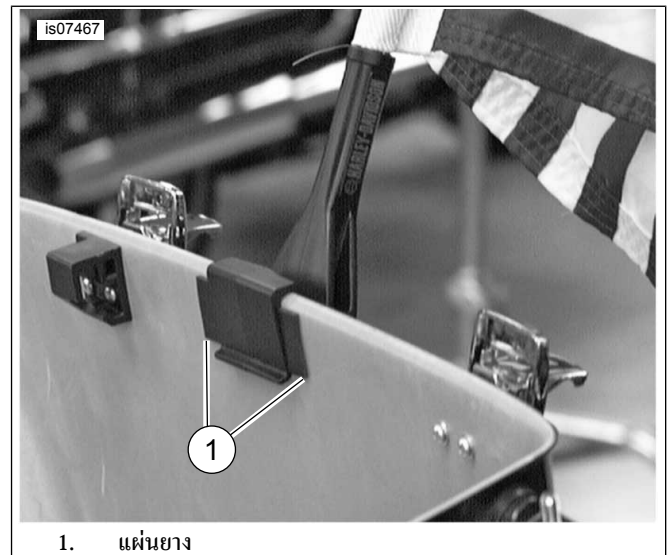
รูปภาพ 2 แผ่นยางที่ติดตั้งกับภายในของ Tour-Pak
