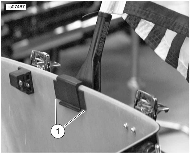
Şekil 2. Tour-Pak'ın İç Kısına Monte Edilmiş Kauçuk Pedler
