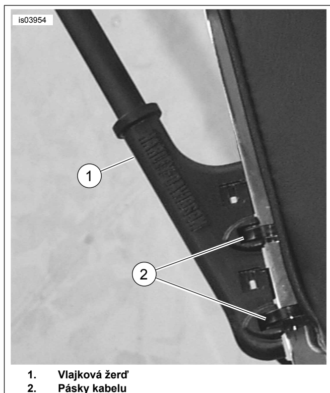
Ilustrace 1. Pohled zvenčí na instalovanou vlajkovou žerď
