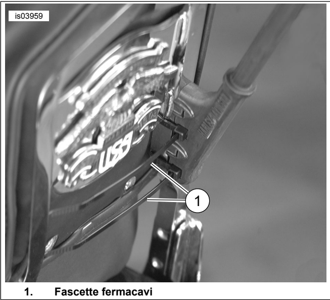
Figura 2. Vista interna dell'asta della bandiera installata
