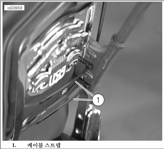
그림 2. 설치된 플러그 마스트의 내부 모습
