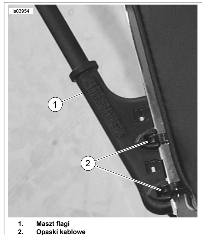
Rysunek 1. Widok zamocowanego masztu flagi od zewnątrz
