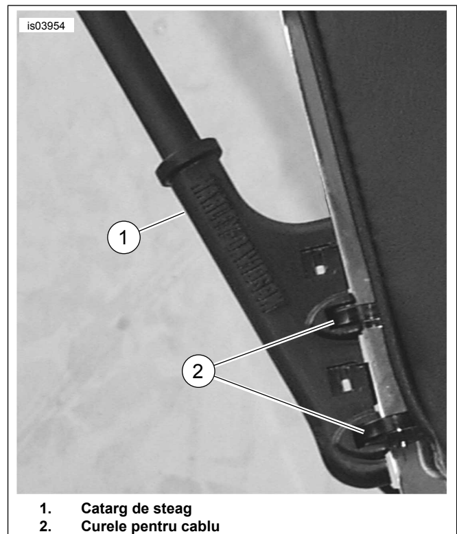
Figura 1. Vedere exterioră a catargului de steag instalat
