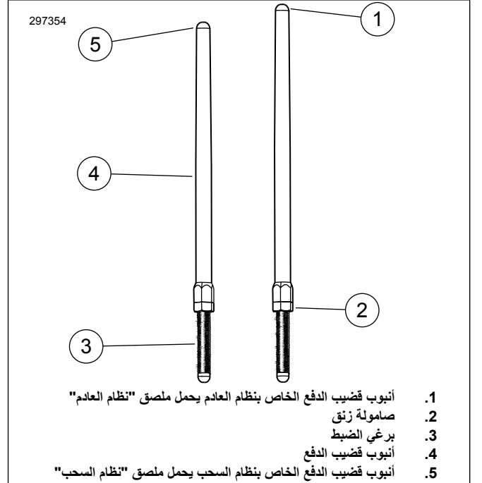
الشكل 1. قضيب الدفع القابل للضبط
